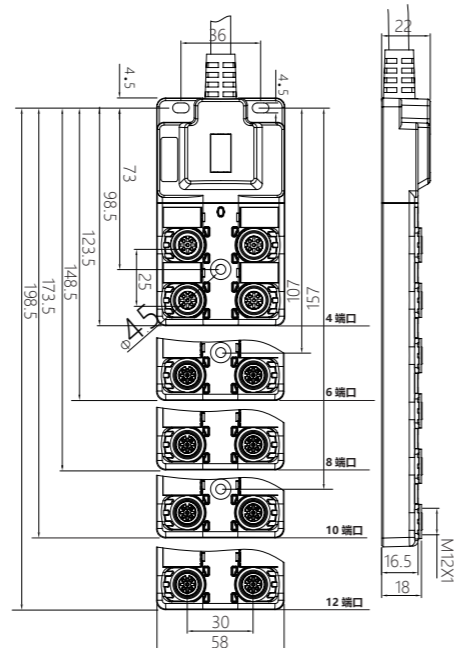
M12 预铸线 -4/6/8/10/12 端口
