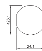
开孔尺寸
